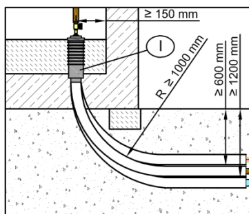
Mehrsparten-Hauseinführung
