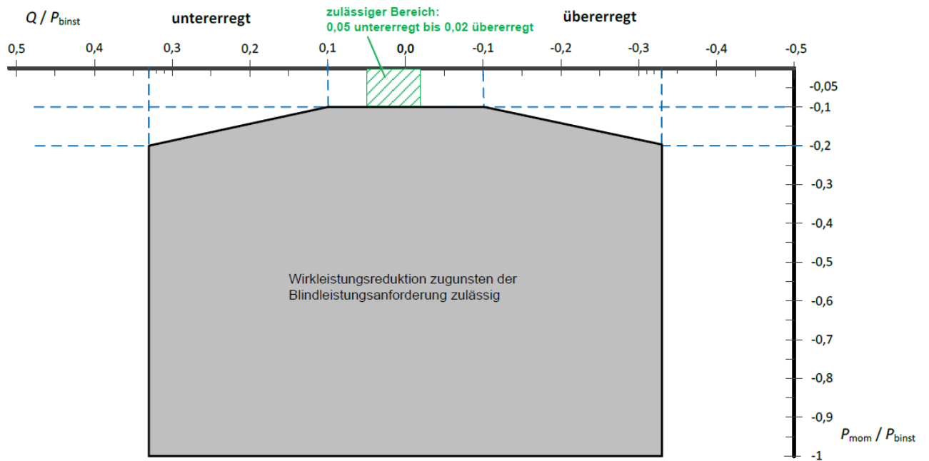
Bild 1 Geforderter Stellbereich der Blindleistung für EZA mit P_{\text{binst}} = P_{rA} \geq 135 \text{ kW} (VDE-AR-N 4110)
