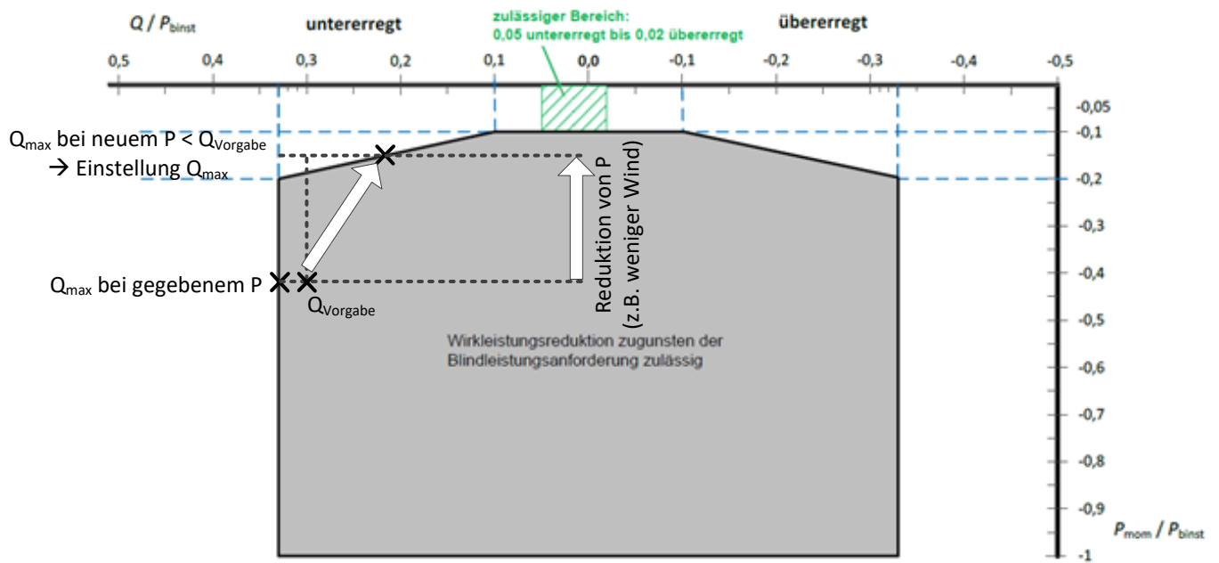
Bild 2 Verhalten bei Überschreitung der Blindleistungsgrenze P durch Wirkleistungsreduzierung ( P_{\text{binst}} = P_{rA} )
