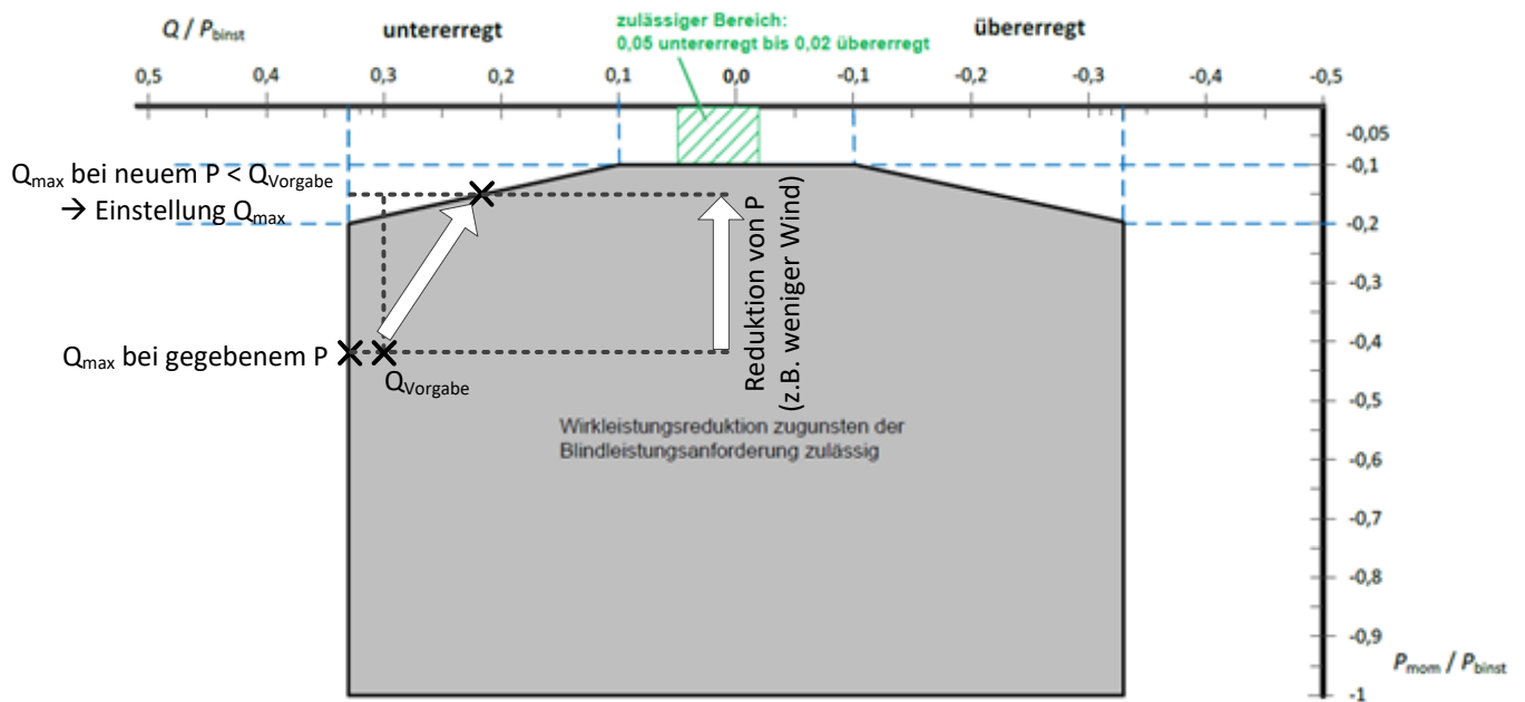
Bild 2 Verhalten bei Überschreitung der Blindleistungsgrenze P durch Wirkleistungsreduzierung ( P_{\text{binst}} = P_{rA} )
