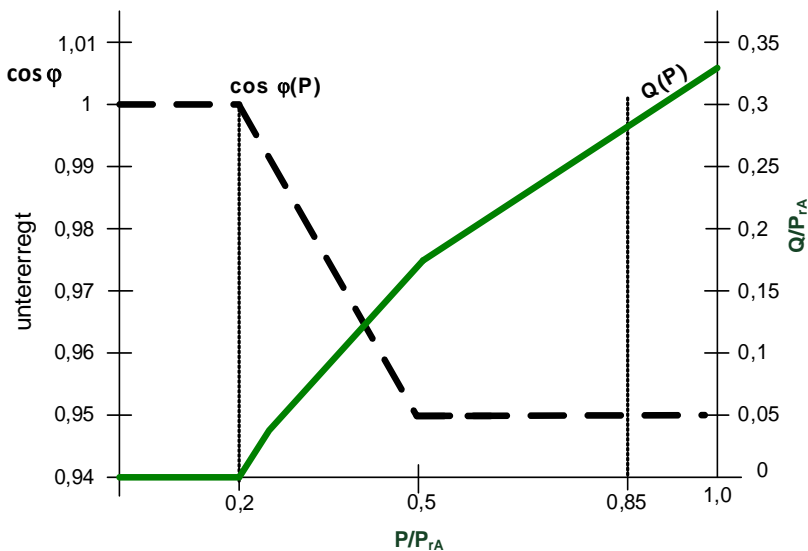
Bild 2 Q = f(P/P_{rA}) -Kennlinie für EZA mit P_{rA} \geq 135 \text{ kW} und Anschluss in den Umspannungsbereichen Königsbrück, Kamenz, Zescha, Kleinsaubernitz, Niesky, Görlitz und Weinhübel
