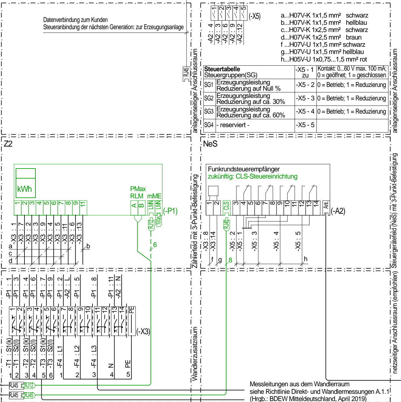
Bild 2 Aufbau Zählerplatz / NeS-Platz (Wandlerrmessung)
