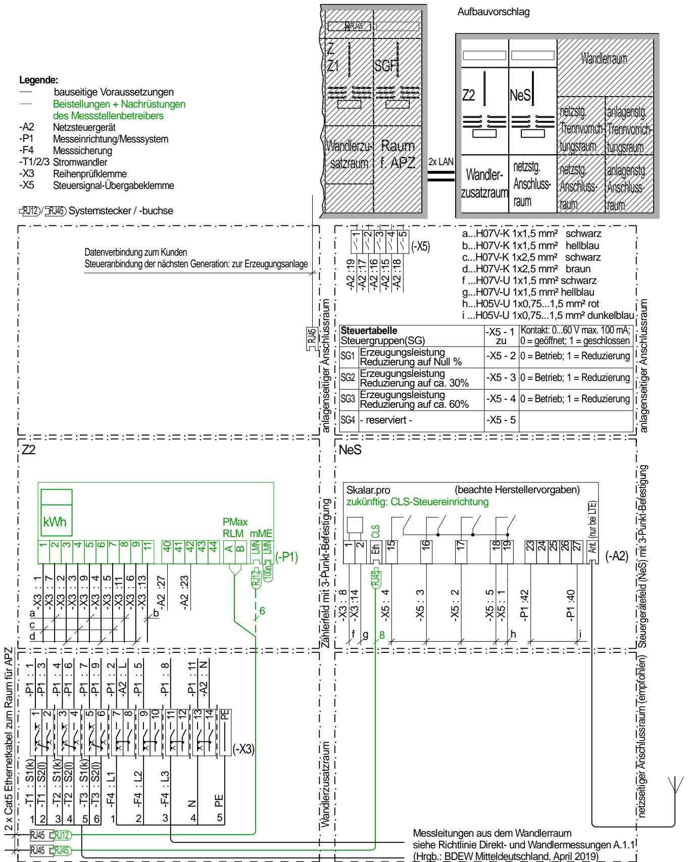
Bild 2 Aufbau Zählerplatz / NeS-Platz Anlagenklasse 1 (Wandermessung)
