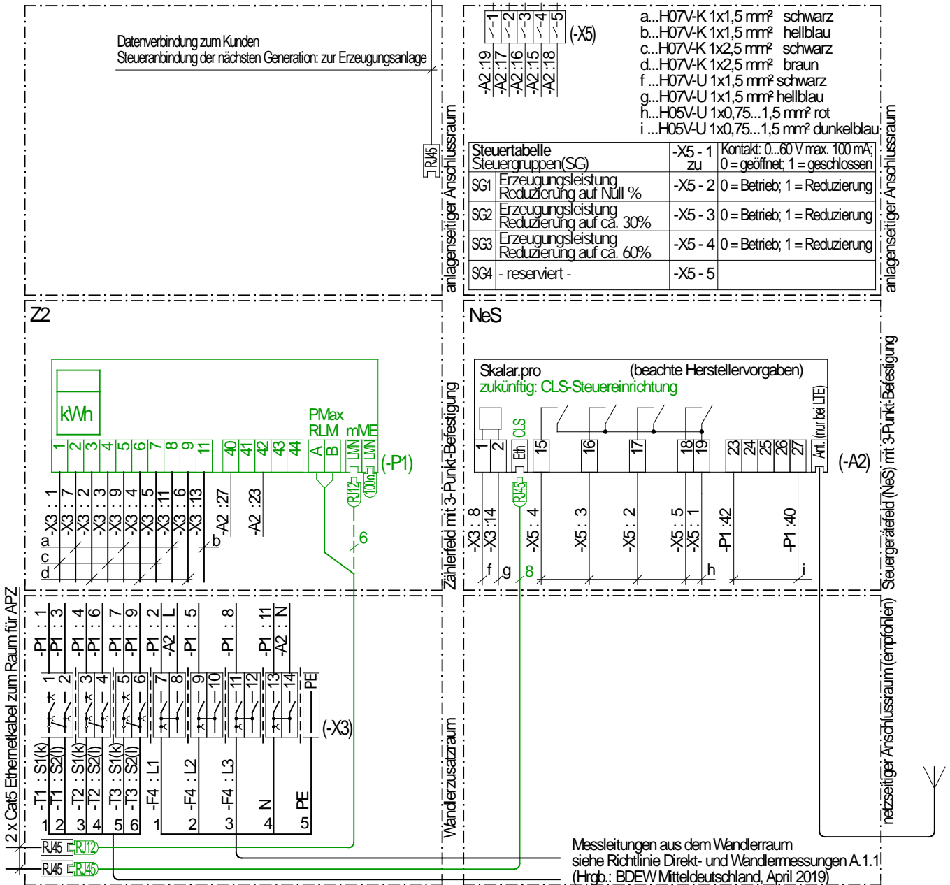
Bild 2 Aufbau Zählerplatz / NeS-Platz Anlagenklasse 1 (Wandermessung)
