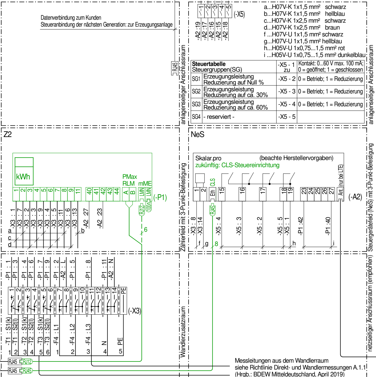
Bild 2 Aufbau Zählerplatz / NeS-Platz Anlagenklasse 1 (Wandermessung)
